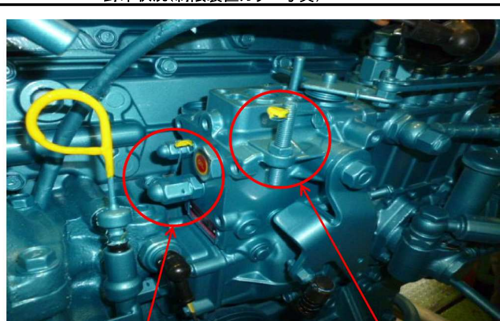
封印状況(制限装置カラー写真)
