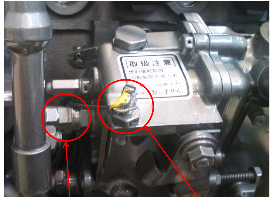
燃料最大噴射量制限装置
