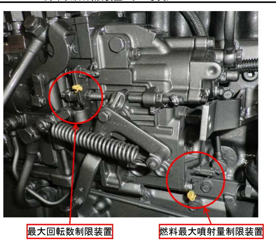
封印状況(制限装置カラー写真)
