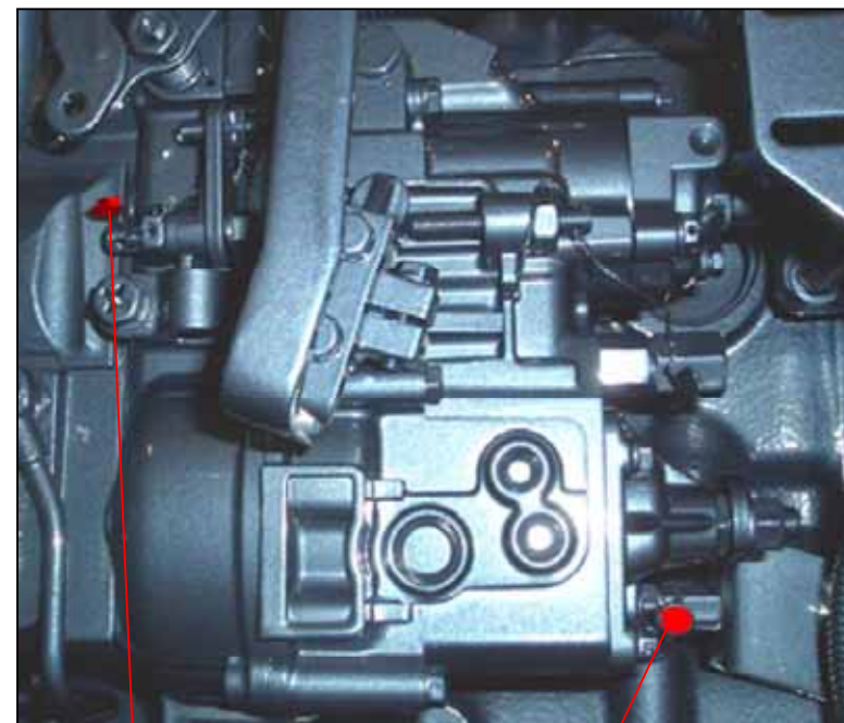
燃料最大噴射量制限装置
