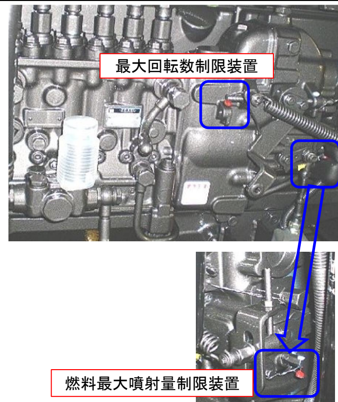
封印状況(制限装置カラー写真)
