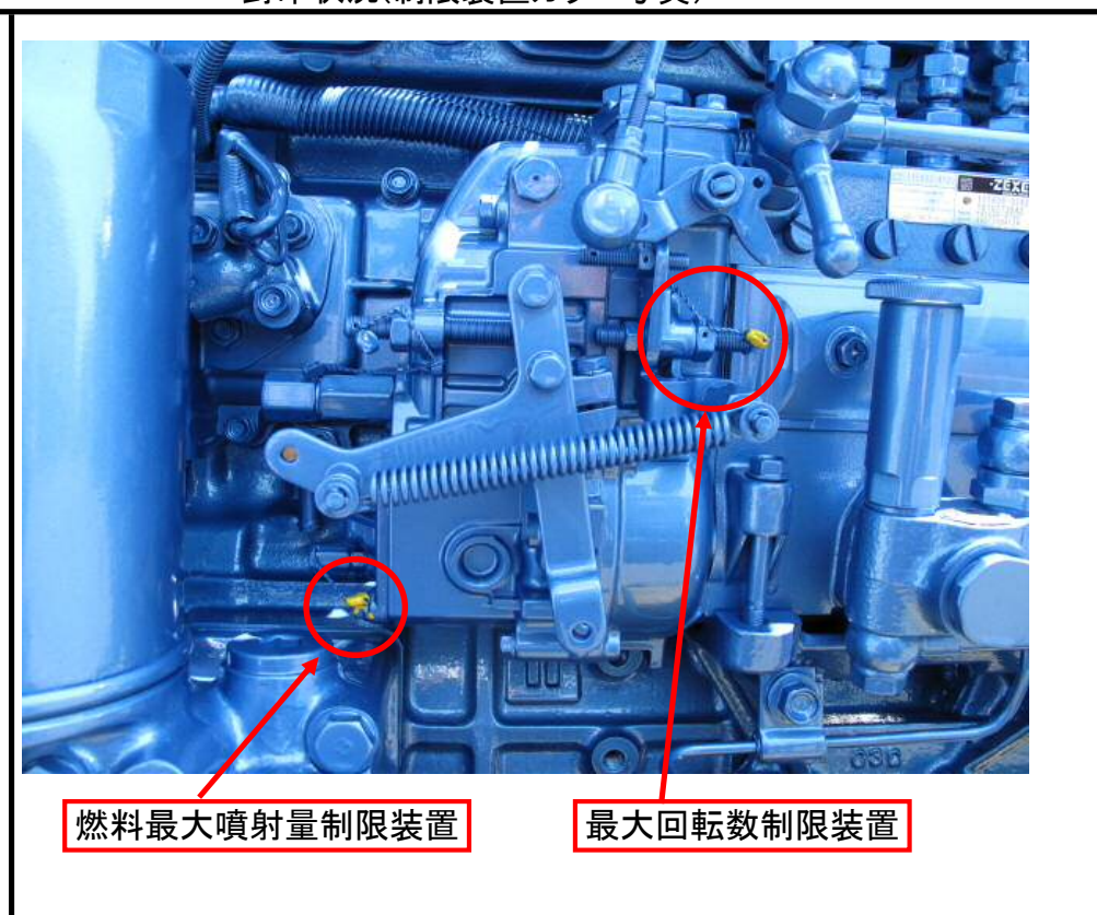
封印状況(制限装置カラー写真)
