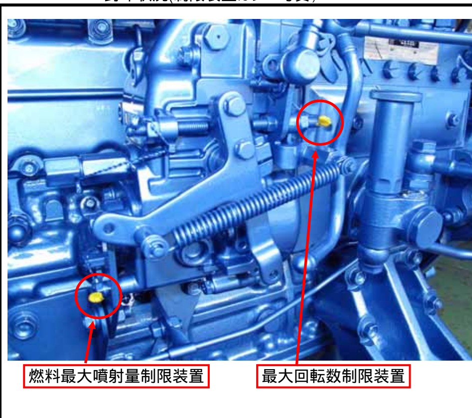
封印状況(制限装置カラー写真)
